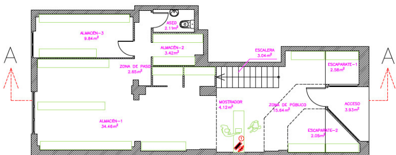
PLANTA BAJA
